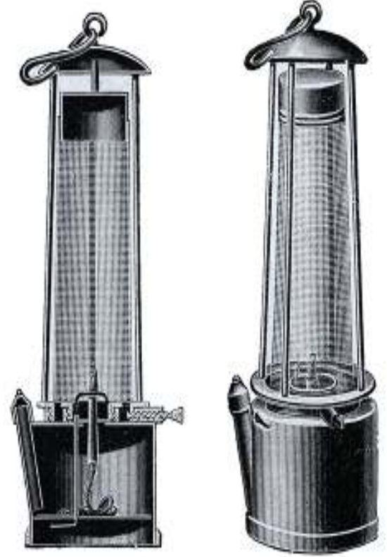
பாதுகாப்பு விளக்கு
