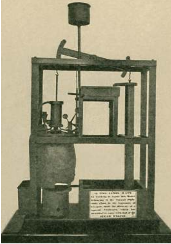
நீராவி இயந்திரம்
